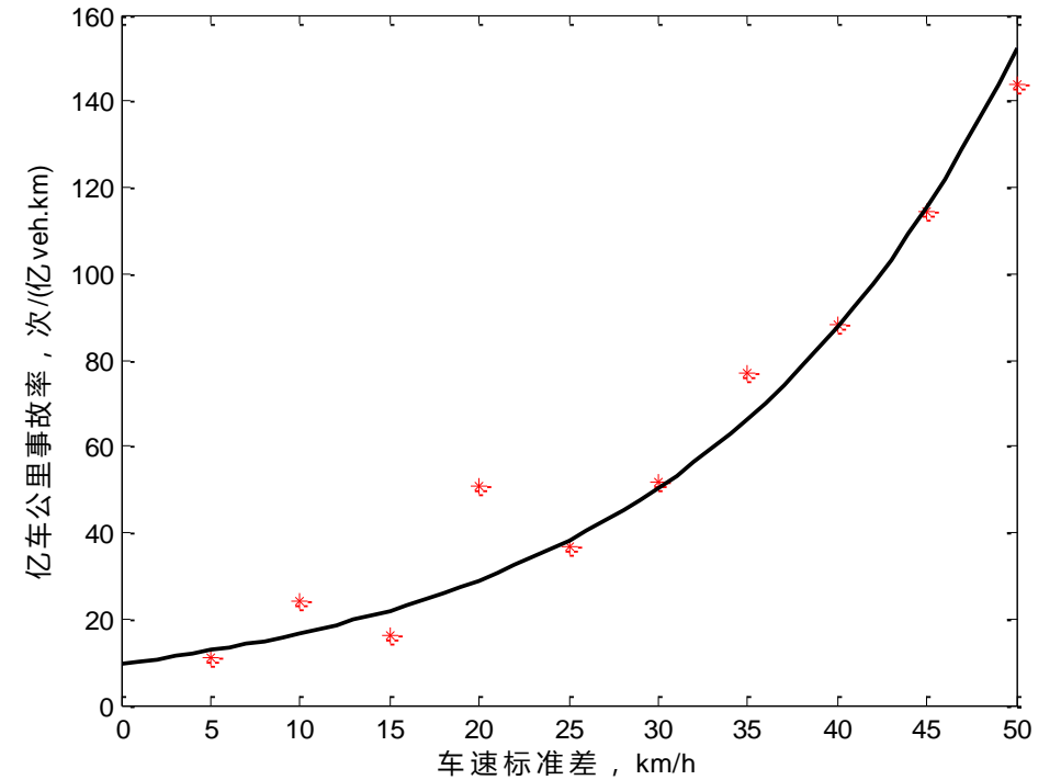
拟合出来的事故率与车速标准差函数图像
